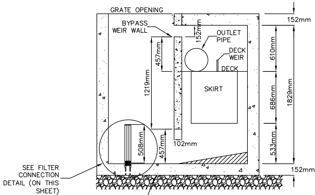
Section View A-A SCALE: 1:30
